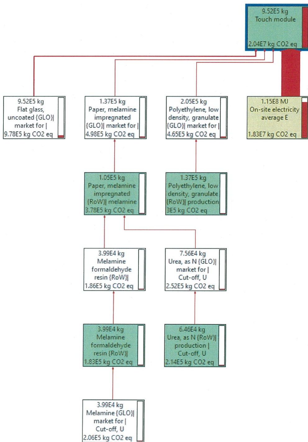
图5.2 touch module1生命周期建模总图
